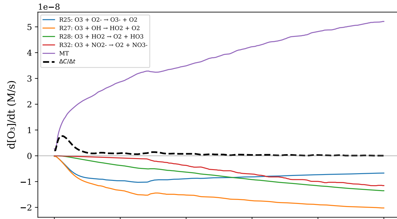
(d) \text{H}_2\text{O}_2
